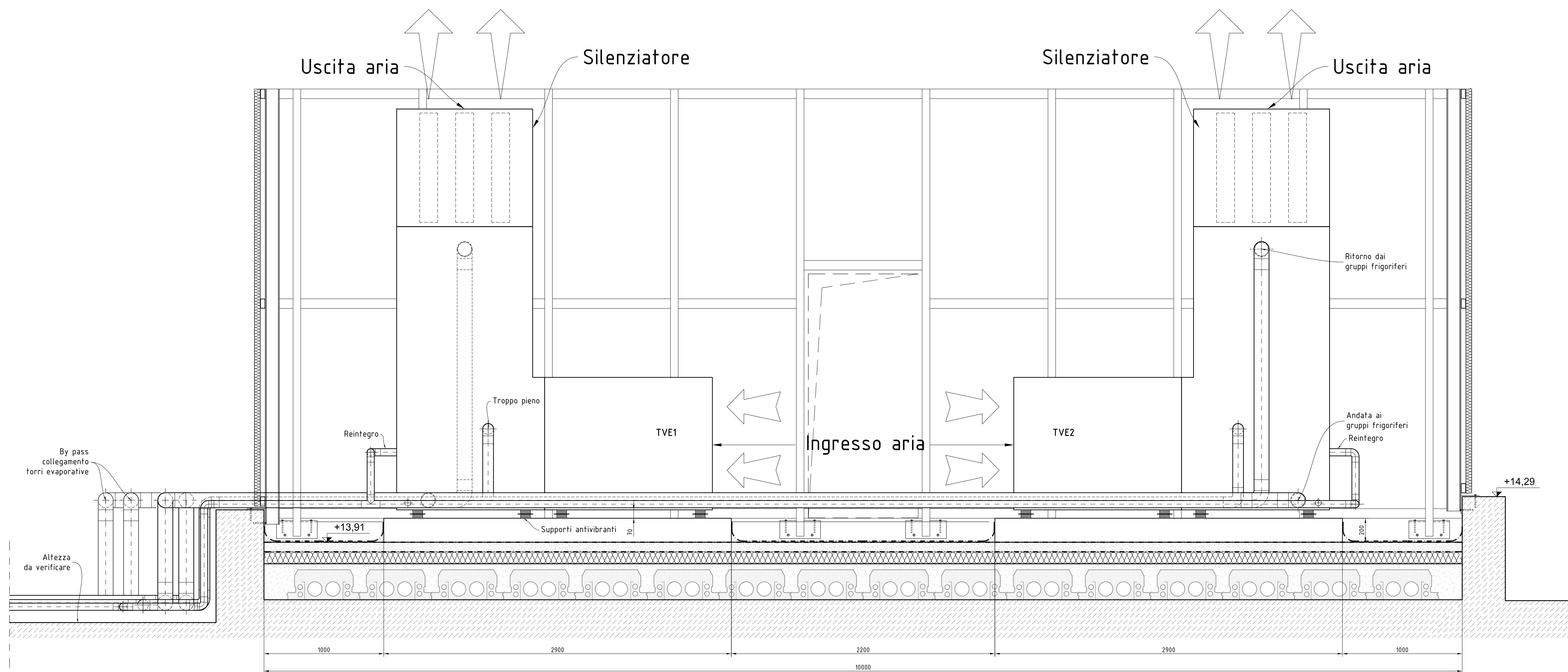
SEZIONE A-A
